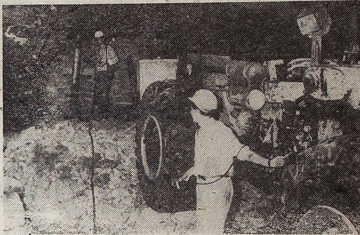
Mgr inż. Lesław Ostapów (z prawej) przy skonstruowanym przez siebie urządzeniu do rozpięcia indywidualnych stojaków hydraulicznych.
