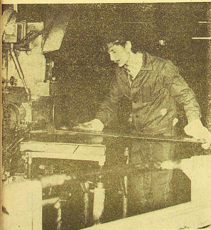
Tak powstają żeberka radiatorów. Przy zgrzewarce Stani- sław Bazak.
