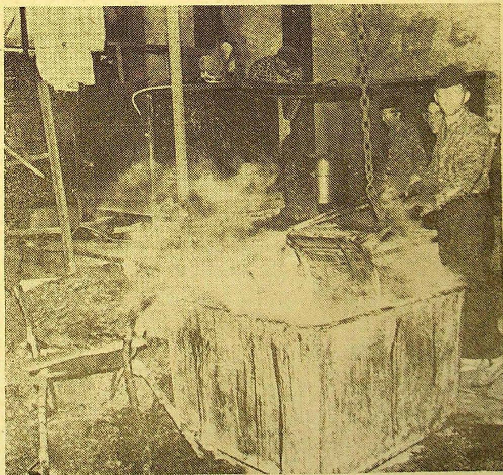
Na tym oddziale praca szczególnie ciężka. W cynkowni obrazek niczym z XIX-wiecznej manufaktury. Technologia na wskroś prymitywna. Przy wannie zatapiające Stanisław Świe- rzewski, Jan Tarakowicz, Zdzisław Durkalec i Roman Popielski.
