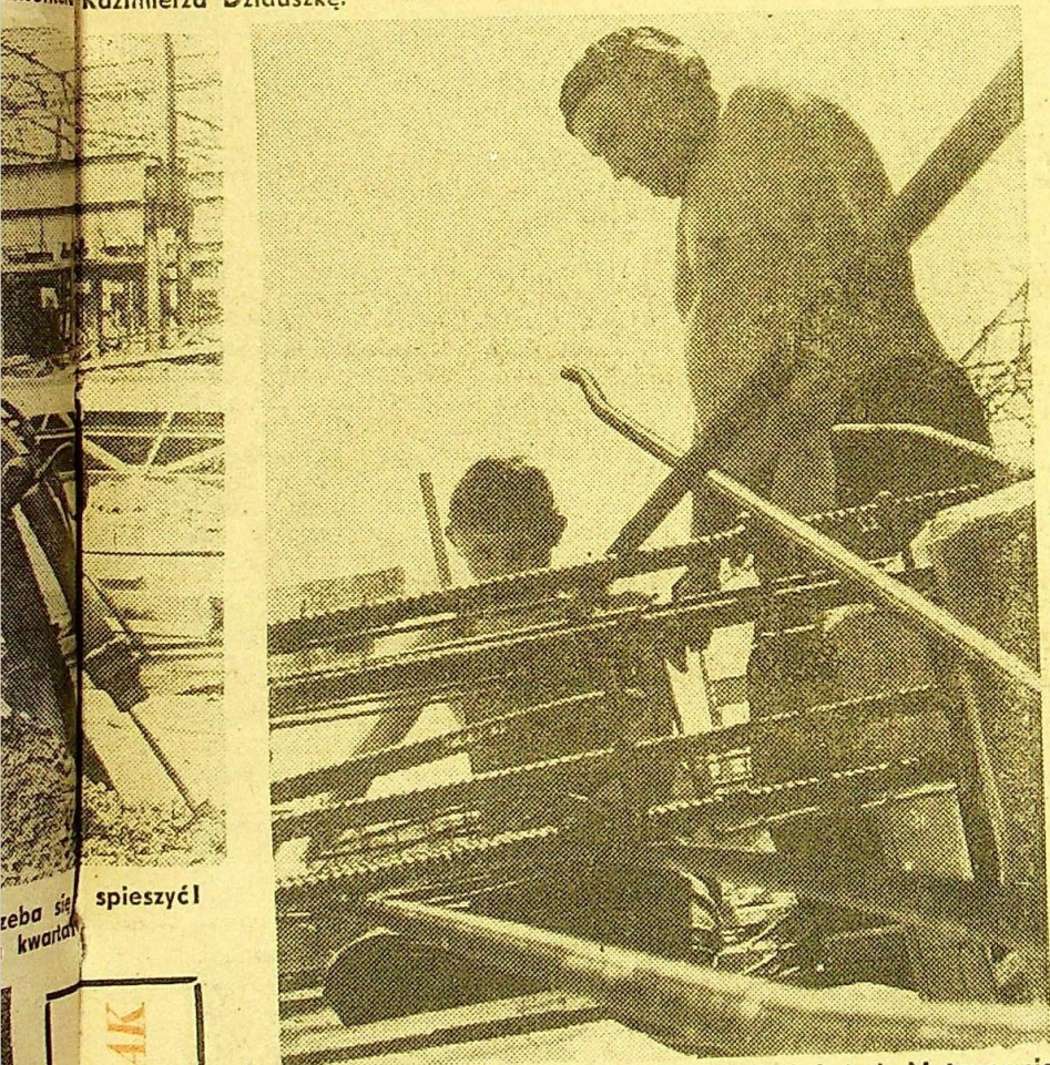
Ramy typu „H” to podstawa konstrukcji hal. Matrycownia będzie miała wymiary 276 x 90 m, a więc zapotrzebowanie na ramy jest olbrzymie. Na zdjęciu Waław Waluśkiewicz z WPBP i Henryk Swirzewski z OHP.
